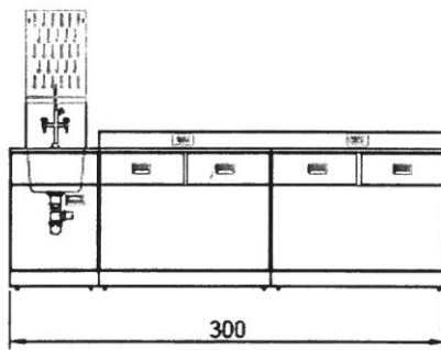
正視圖
