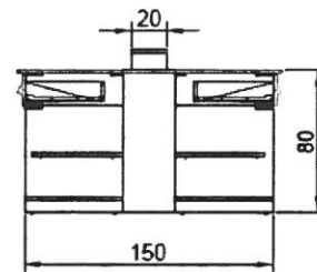
側視圖
